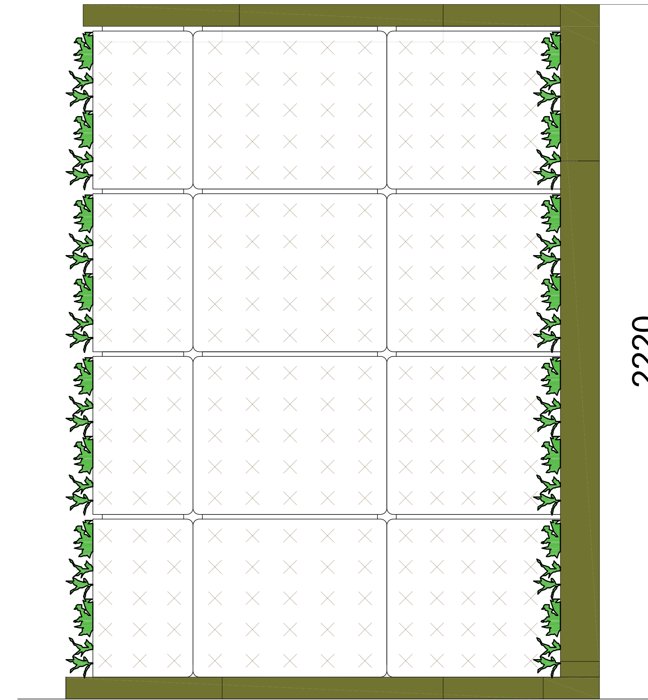
Aanzicht B
