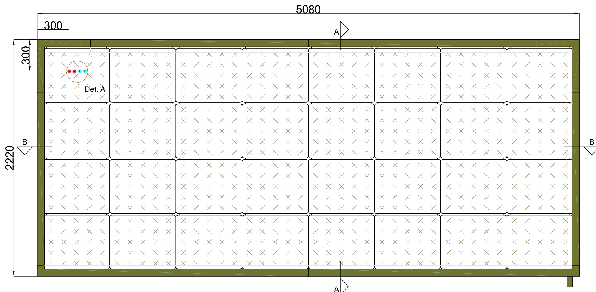
Vorderansicht
