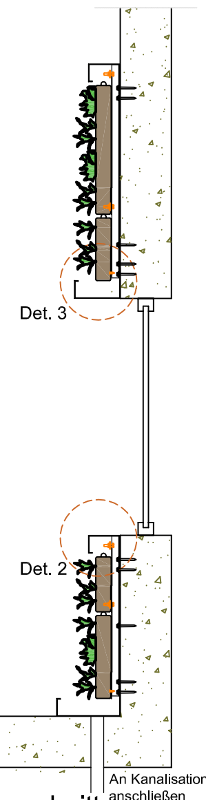
Querschnitt A-A
