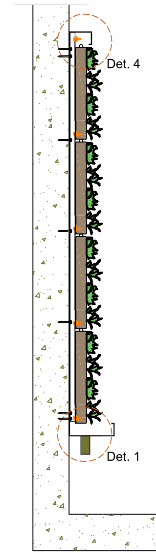
Querschnitt A-A
