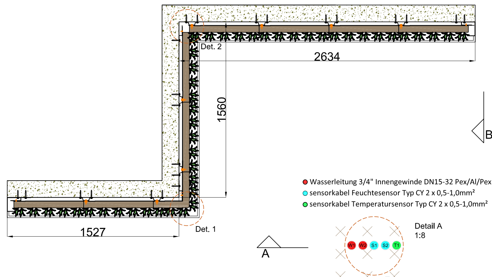
Ansicht A.
