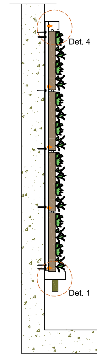
Querschnitt A-A
