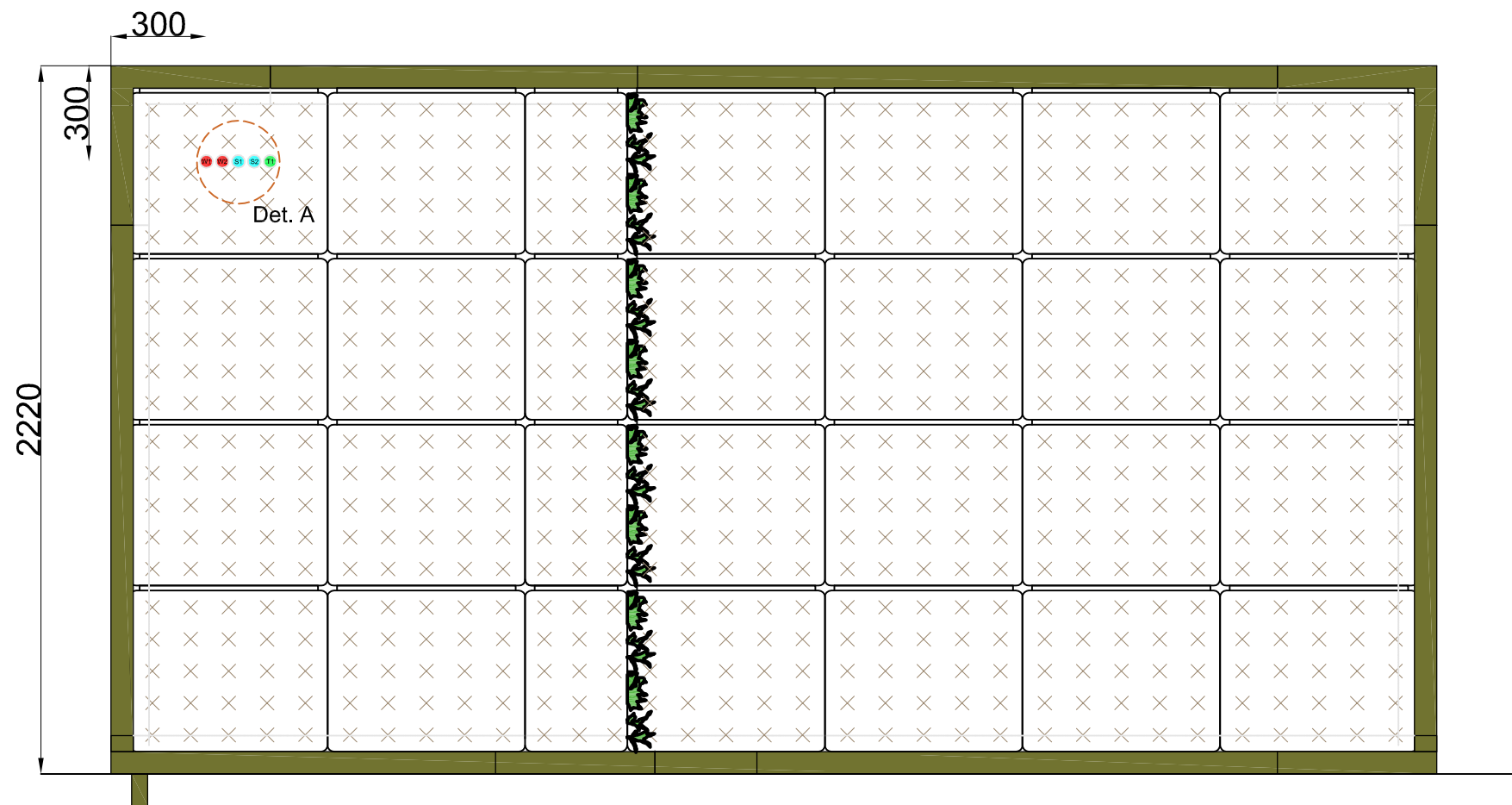
Ansicht A.
