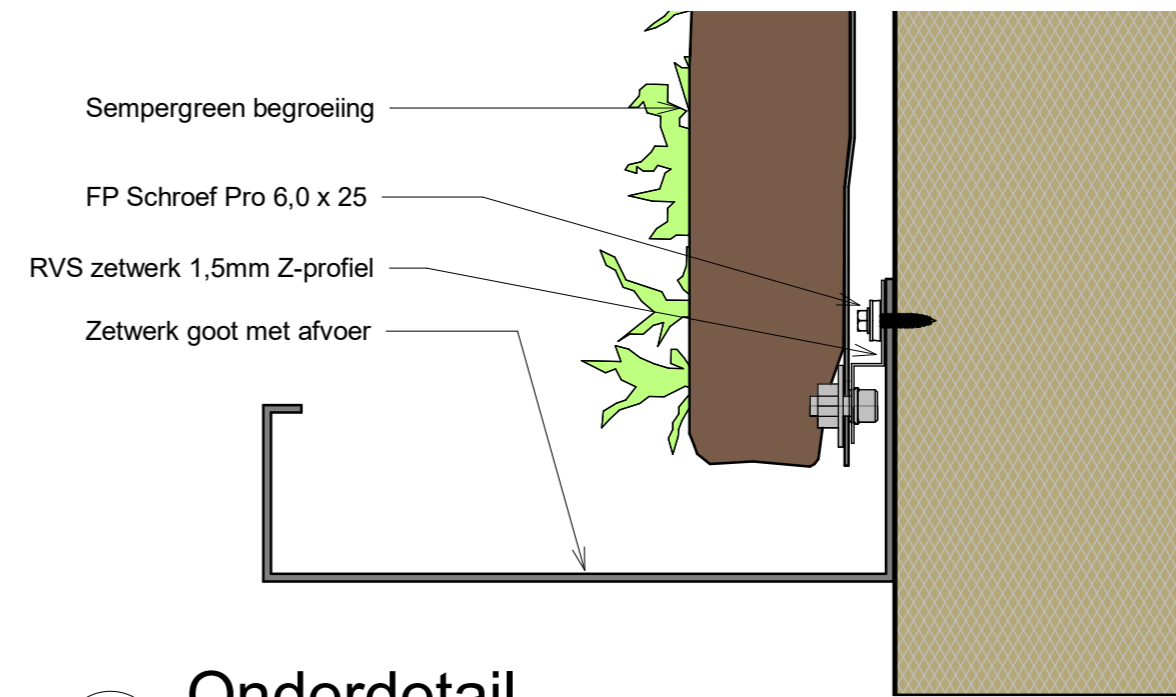
2 Bovendetail 1 : 3
